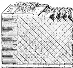
Fig. 508. Structura reticulata.
